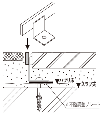
a:ハイタイプ(High type) ステンレスヘアライン
